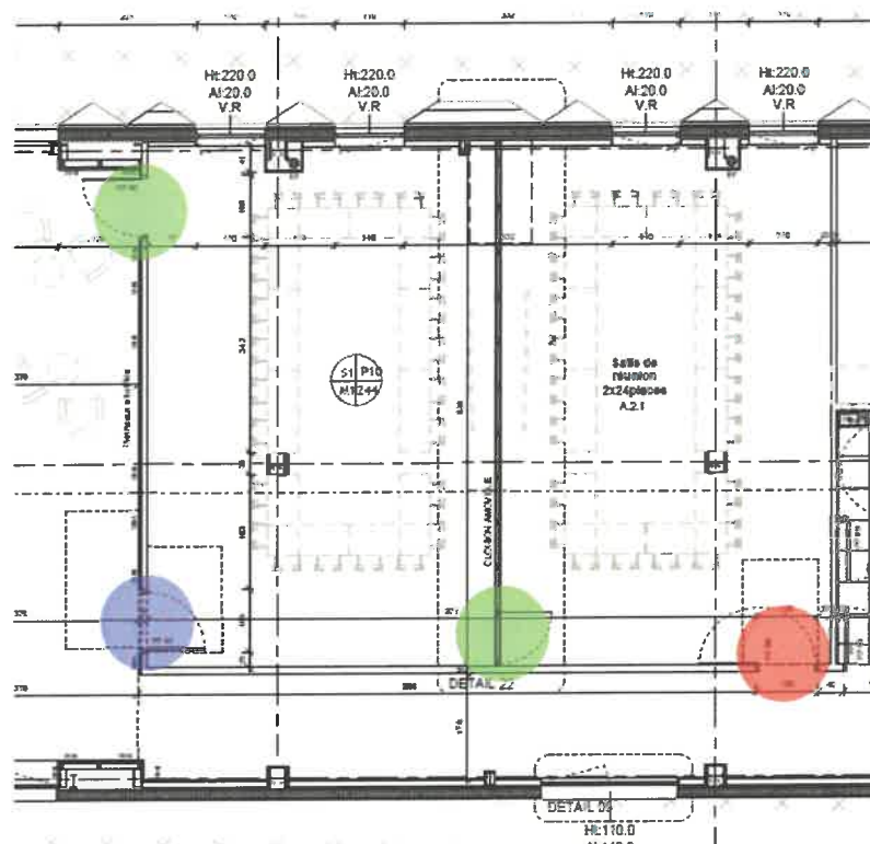
Figure 5 : Défauts de mise en œuvre des blocs-portes – salles de réunion RDC
