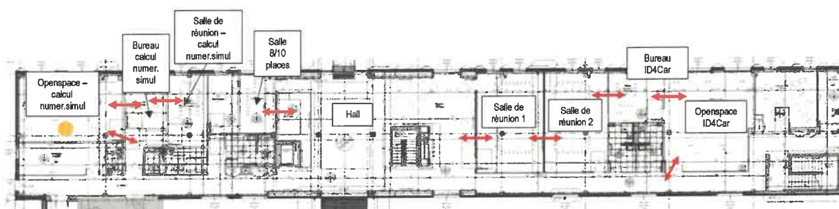
Figure 1 : Mesures acoustiques réalisées - RDC
